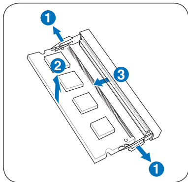
移除内存条
