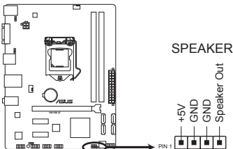
Connecteur pour haut-parleur système de la H61M-E
