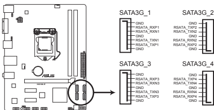
Connecteurs SATA 3Gb/s de la H61M-E
