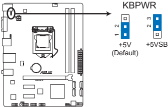
Jumper de mise en route via clavier de la H61M-E
