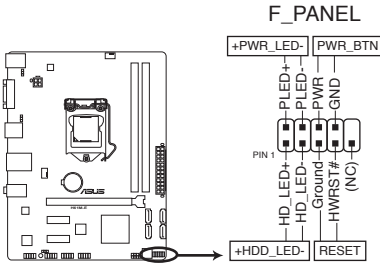
Connecteurs panneau système de la H61M-E
