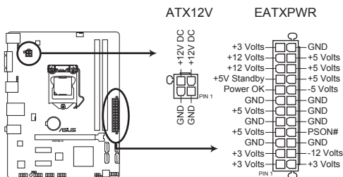
Connecteurs d'alimentation de la H61M-E
