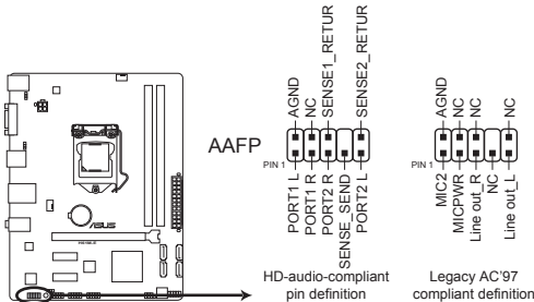
Connecteur pour port audio en façade de la H61M-E
