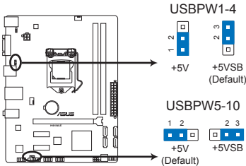
Jumper de mise en route via USB de la H61M-E
