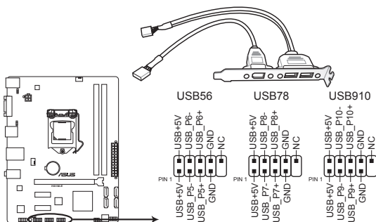
Connecteurs USB de la H61M-E
