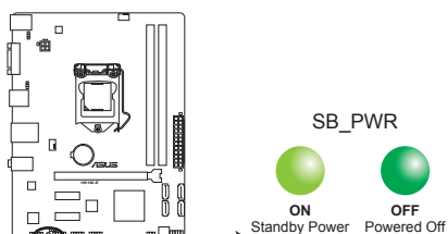
Voyant d'alimentation de la H61M-E
