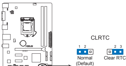
Jumper d'effacement de la mémoire RTC de la H61M-E
