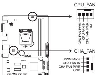
Connecteurs de ventilation de la H61M-E
